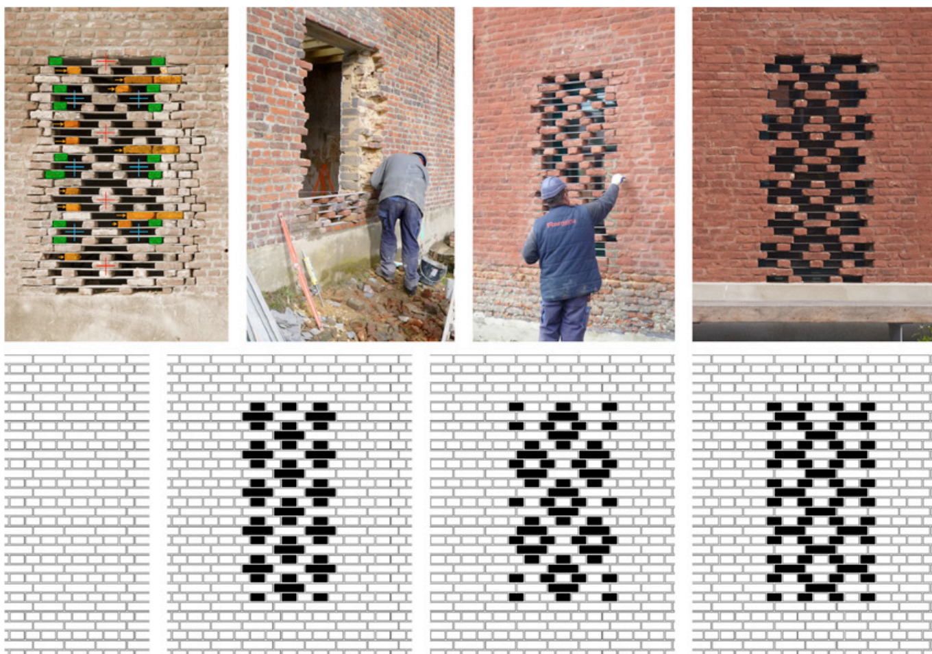
2. Les claustras de la cité des Électriciens, réalisation et représentation géométrale. © Dessins et photos Lucas Monsaingeon, Philippe Prost / AAPP architectes.
